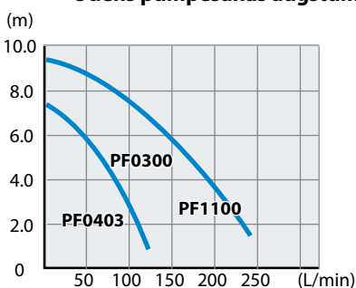
Ūdens pumpēšanas augstums un jauda
