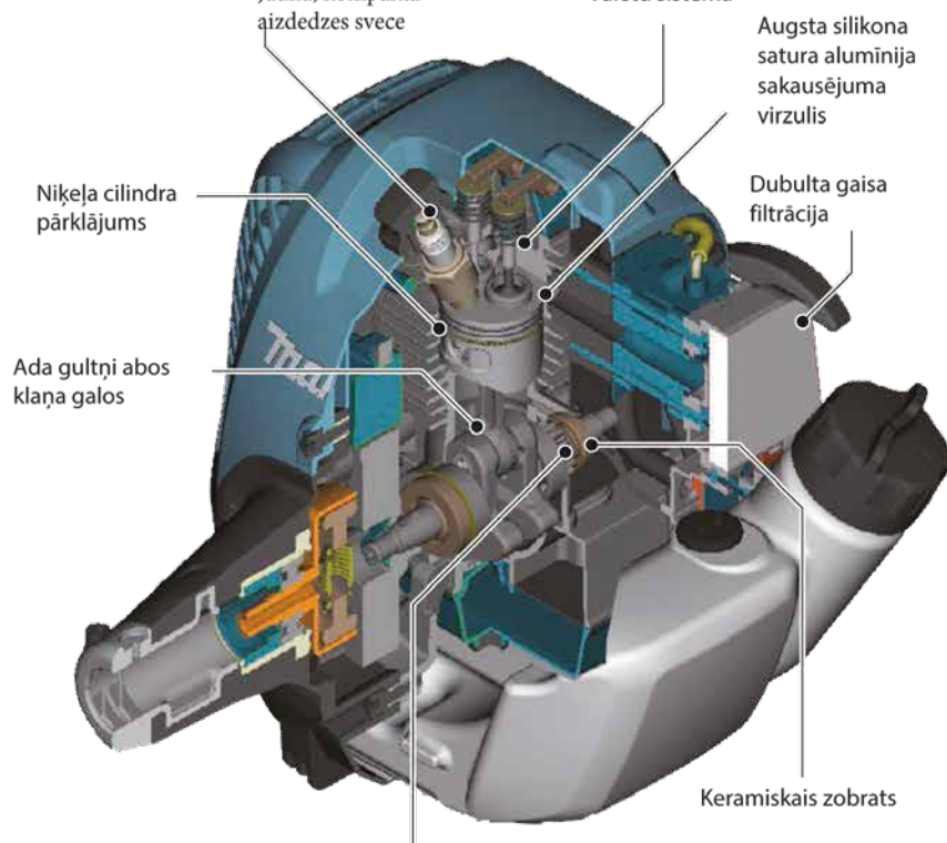
Vārstu sistēma
